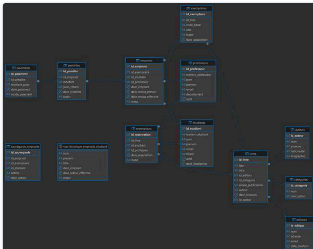
Diagramme Entité-Relation final
